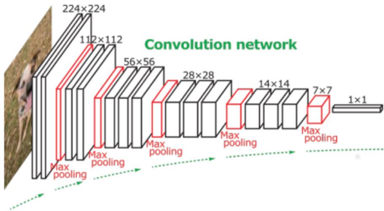
VGG
