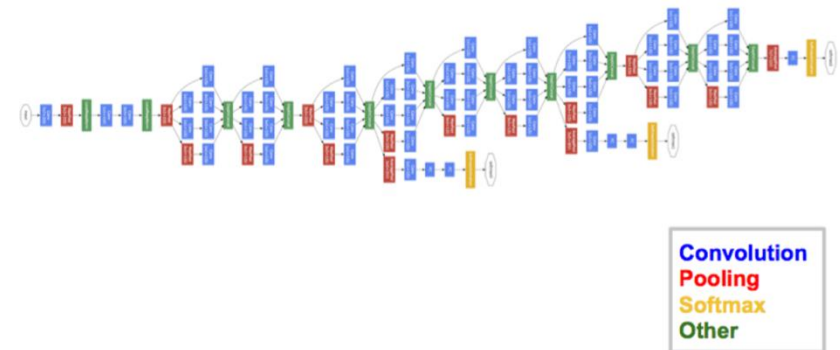
GoogLeNet
